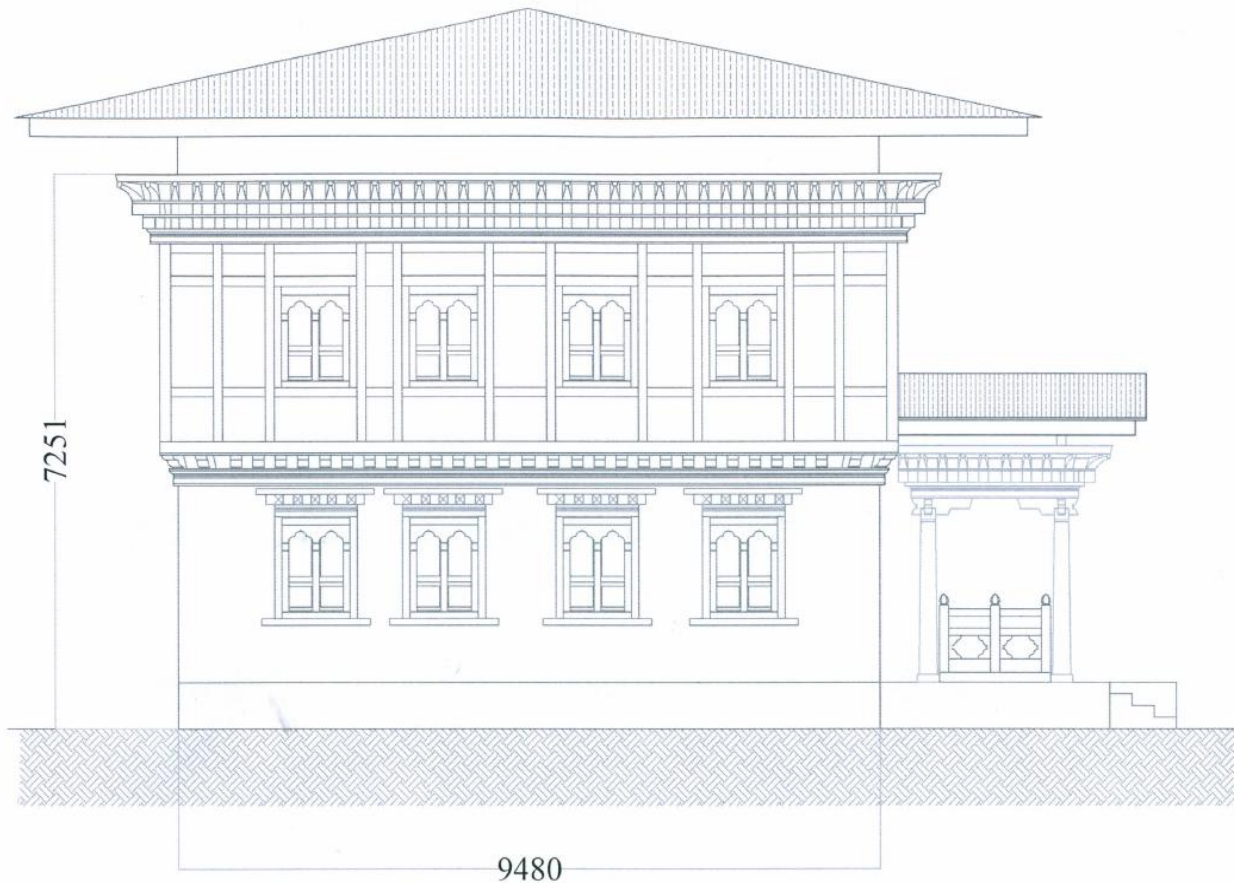
ELEVATION B
